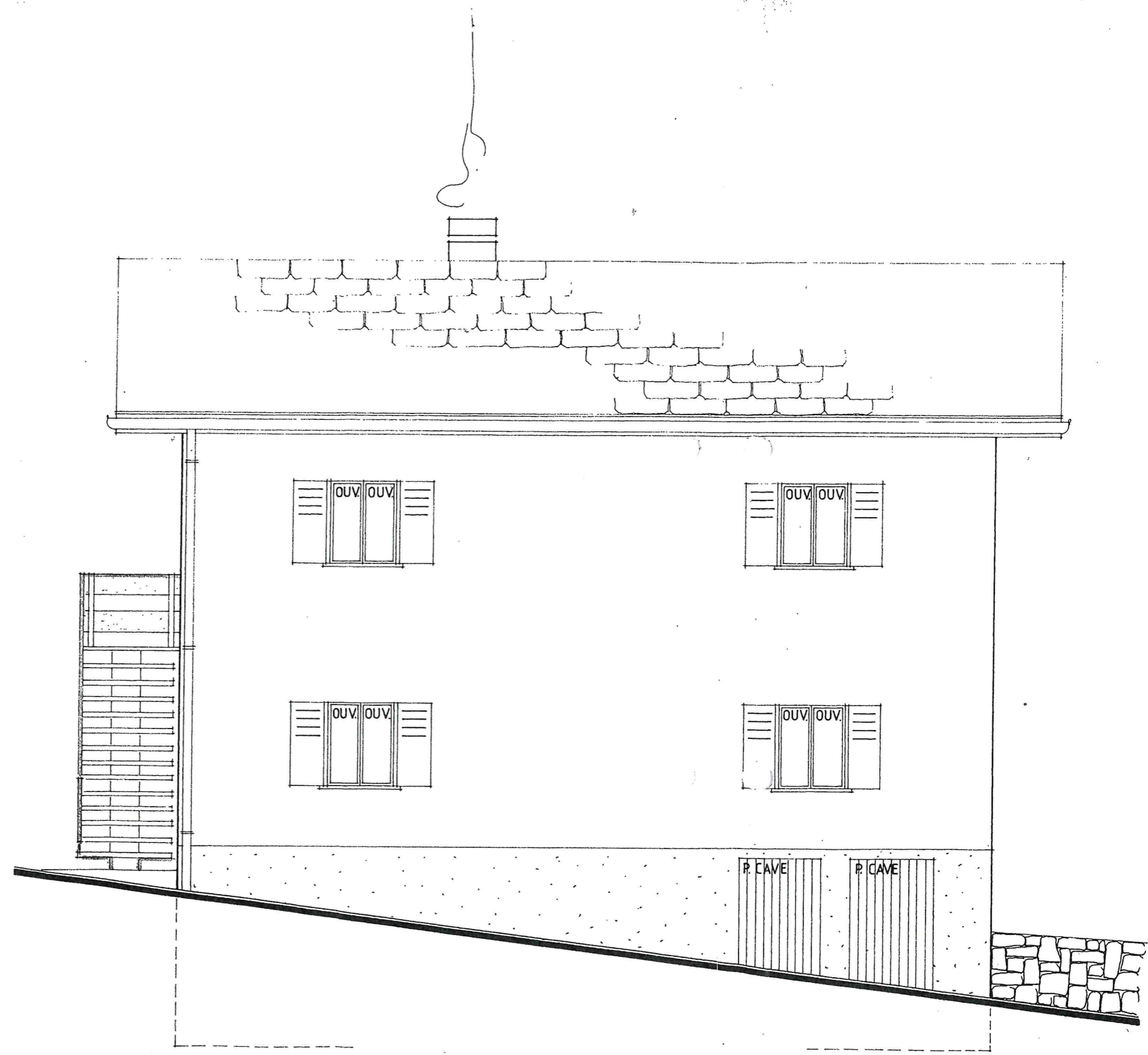
FACADE NORD
