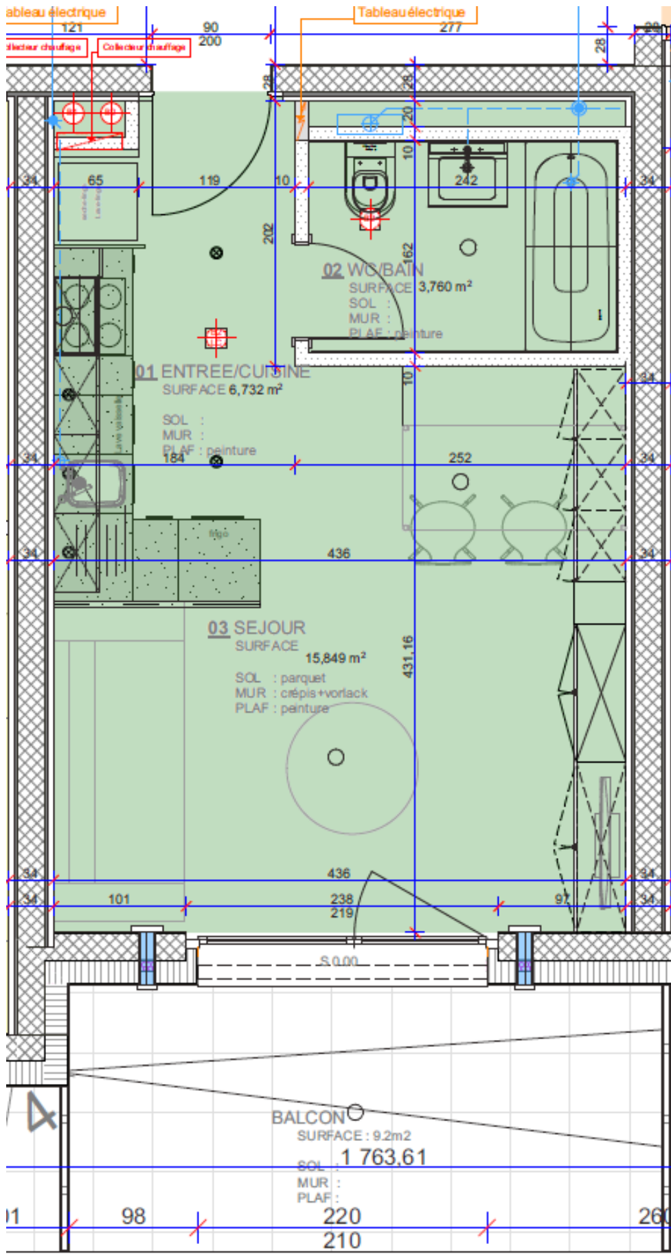
Figure 1.10 : Plan de l'étage d'un appartement (d'après [10]).
