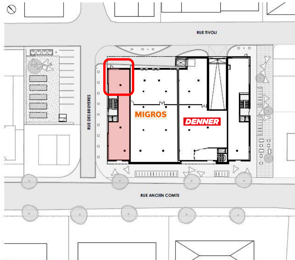
Situation Lot1 - rez-de-chaussée 1:500
