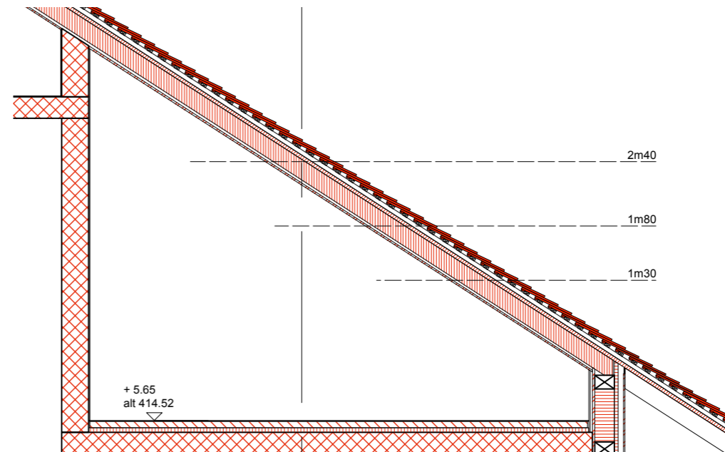
Coupe sur salle de bain 1 1:50e
