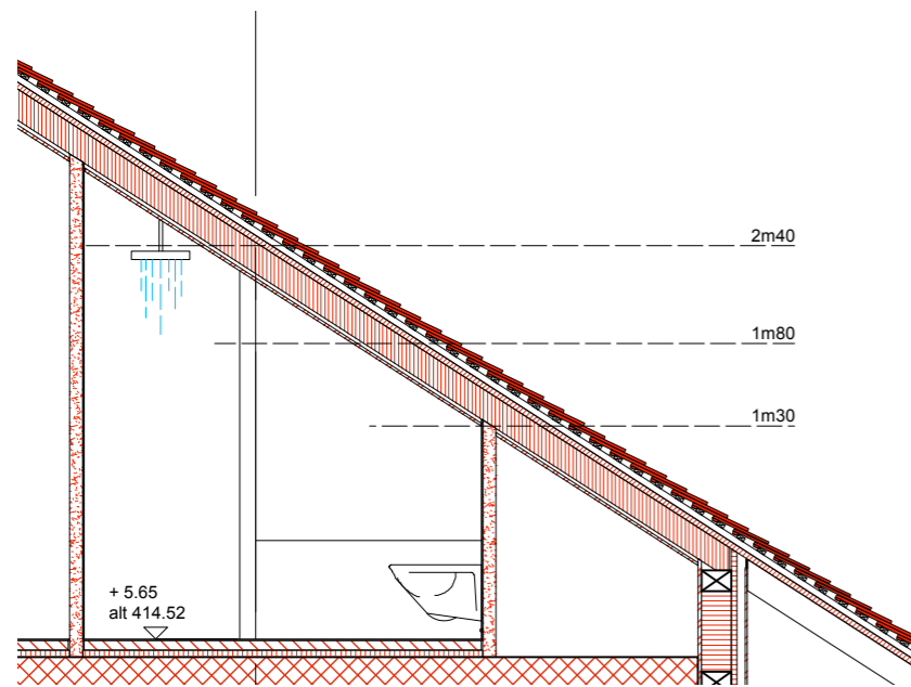
Coupe sur salle de bain 1 1:50e
