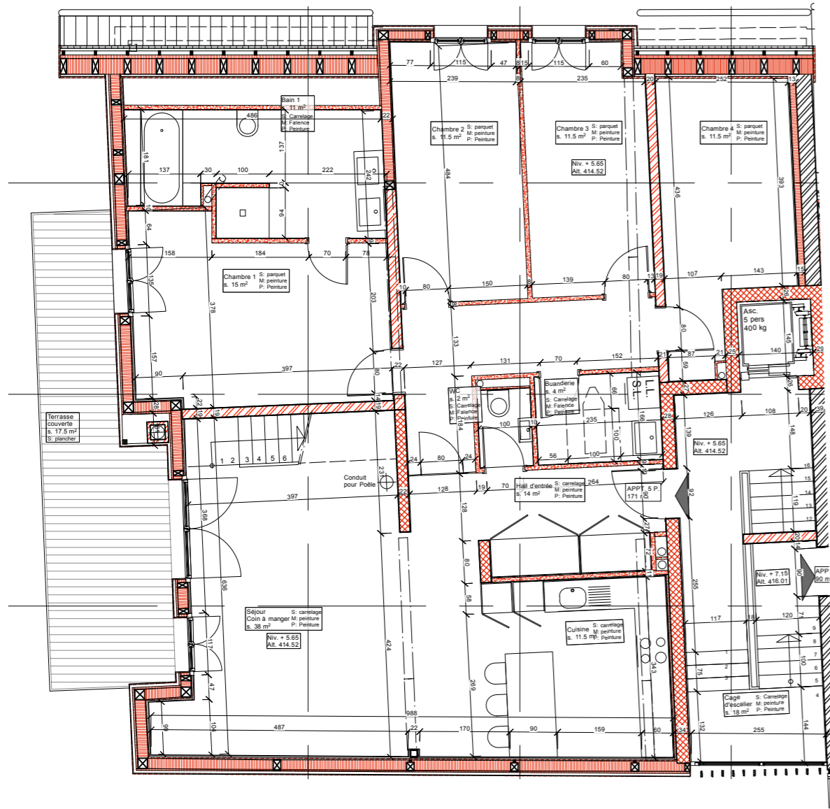
2eme etage 1/100
