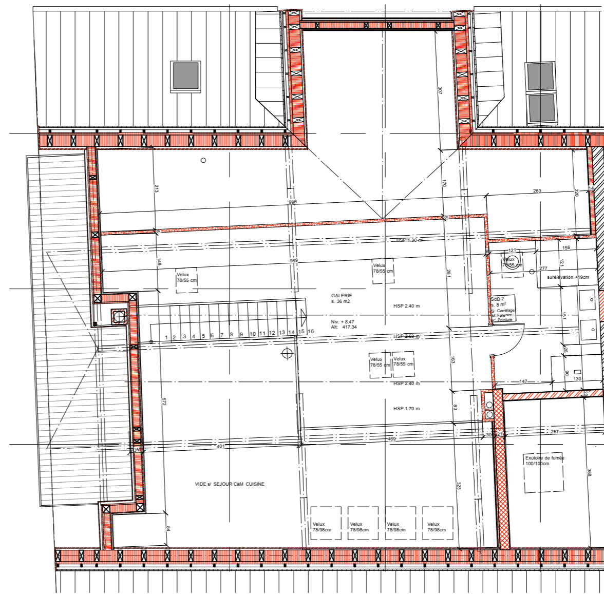
Combles 1/100
