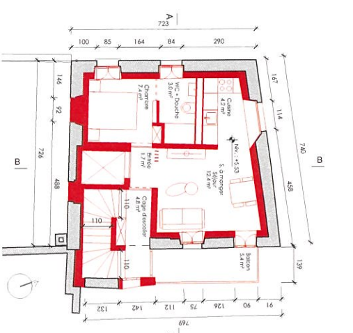
Plan de l'étage 2
