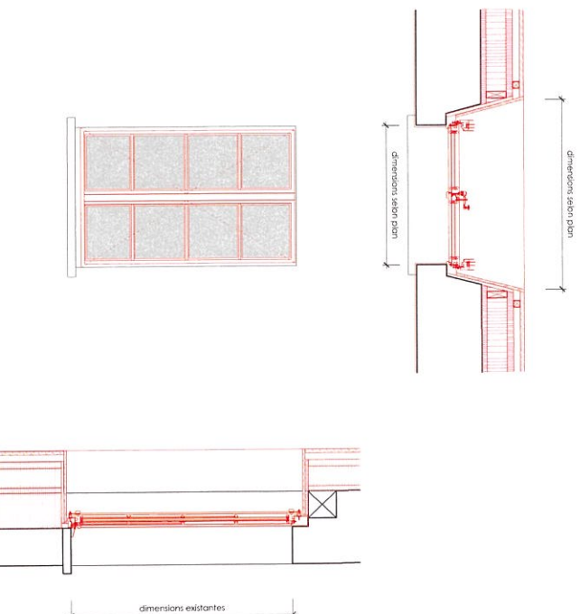
Détails de principe fenêtre 120
