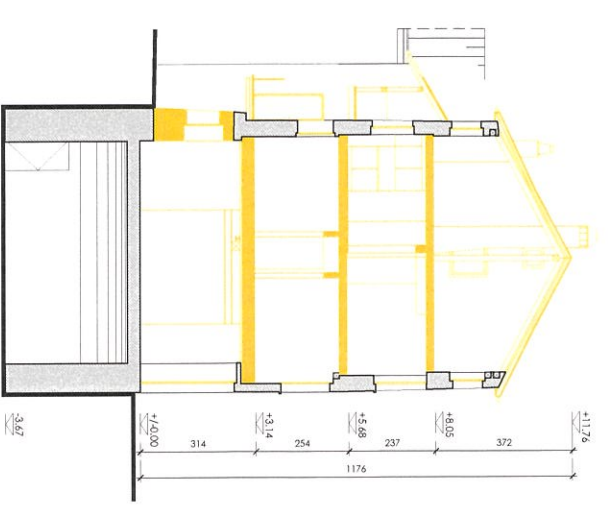
Coupe AA
