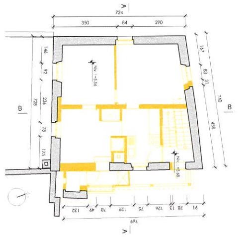
Plan de l'étage 2
