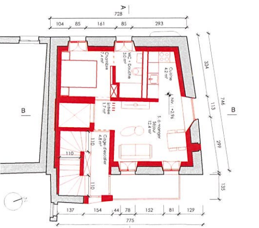
Plan de l'étage 1
