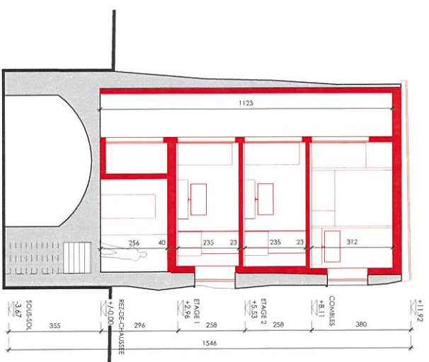
Coupe BB
