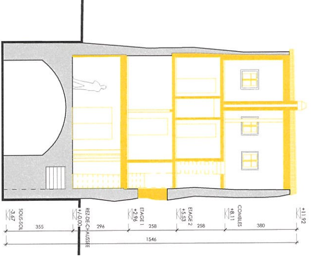
Coupe BB
