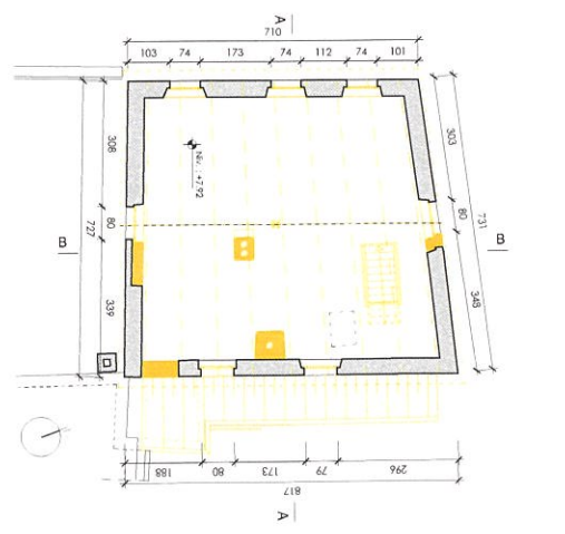
Plan de l'attique
