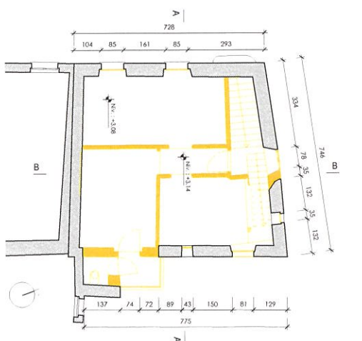
Plan de l'étage 1
