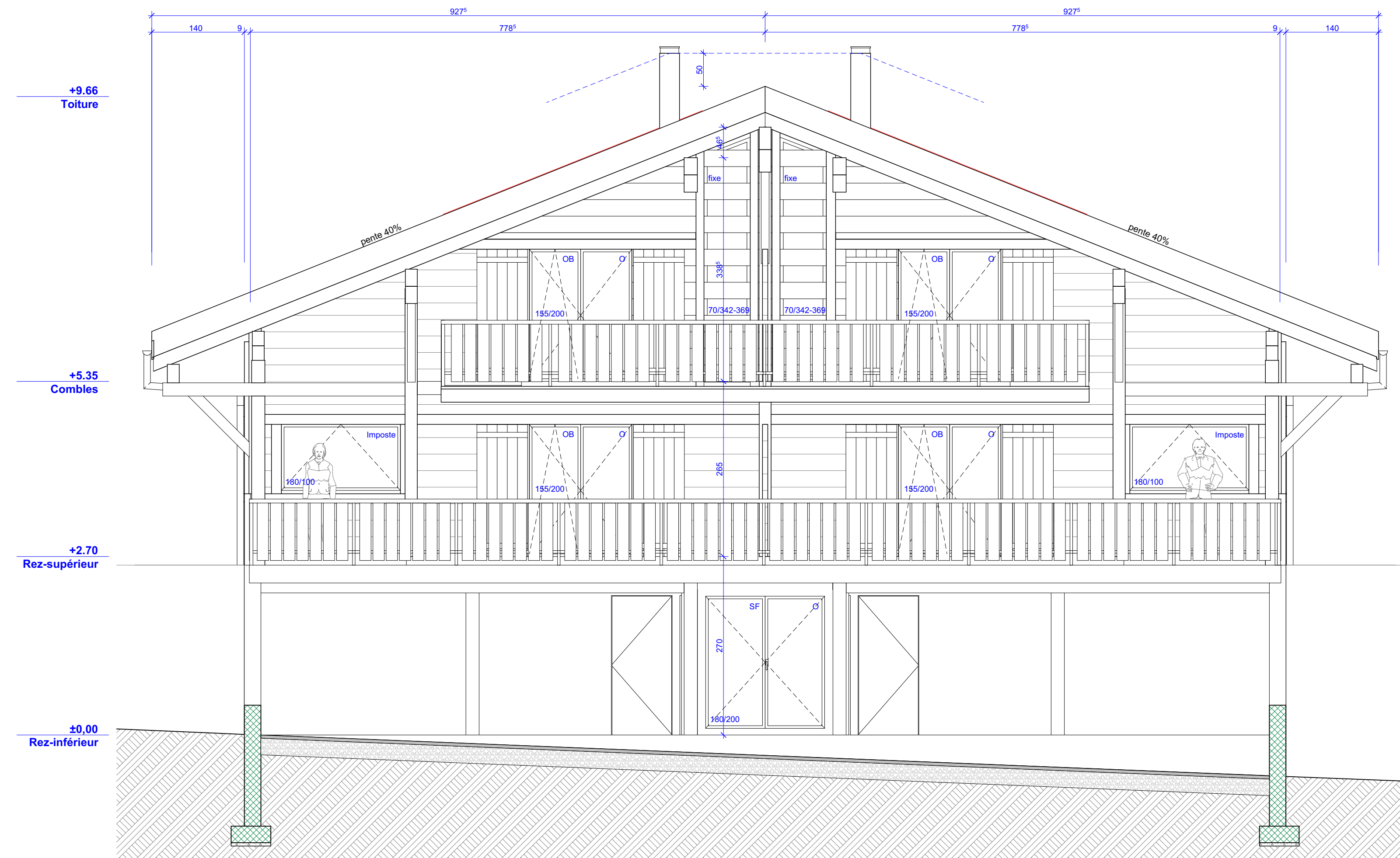
Façade Sud-Est
