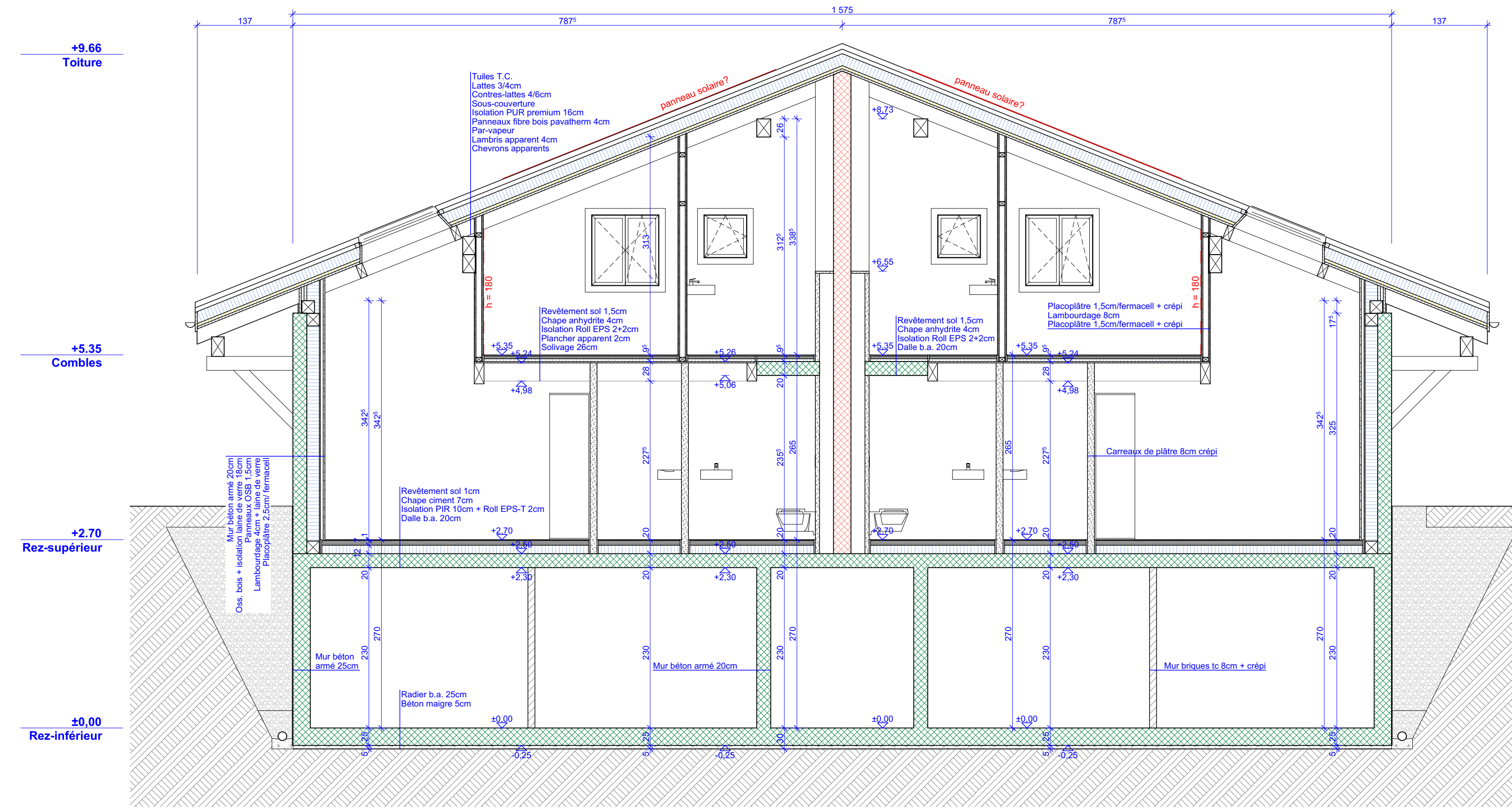
Coupe C-C
